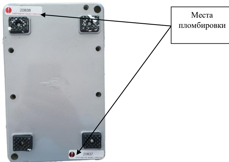
Рисунок 1 – Общий вид мегаомметров
