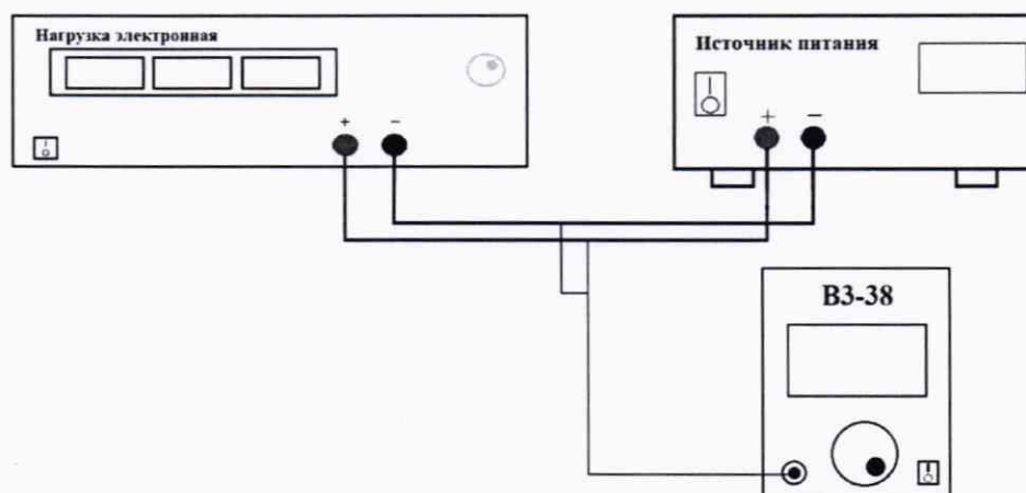
Рисунок 3 – Схема соединения оборудования
